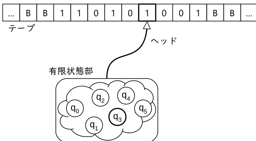
図: チューリングマシンの概念図
